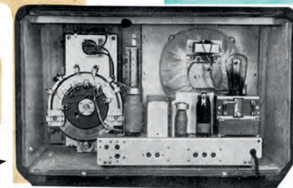
Wnętrze radioodbiornika Automatic
